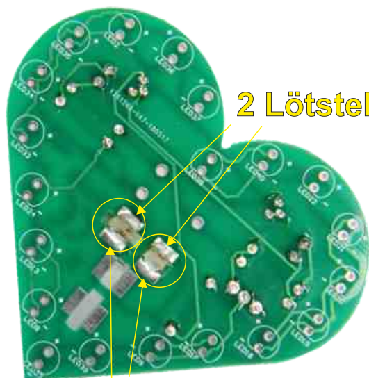
2 Lötstellen
